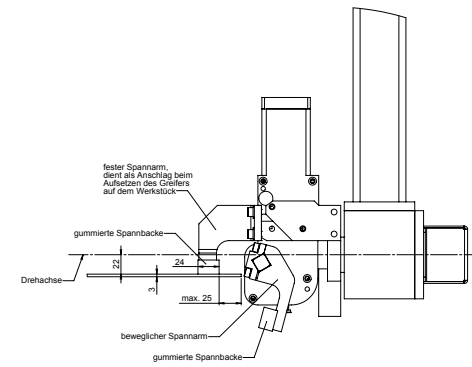
DETAIL Z MAßSTAB 1 : 2
